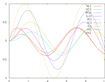
Figura 3: Sistema a. resultados del con fuente de voltaje sinusoidal
