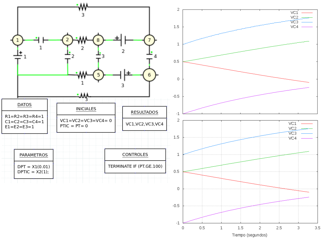
Figura 6: Sistema c. (Izq.): Diagrama y resultados : 2 loops capacitivos, en color verde. (Der. Arr.): programa desarrollado (Der. Aba.): SCEPTRE, con condiciones iniciales ajustadas.
