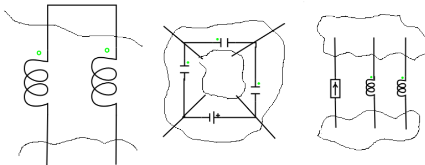
Figura 1. (Izq.): Dos bobinas en serie son un cut-set. (Centro:) Loop de tres condensadores y una fuente de tensión (Der.): Cut-set de dos bobinas y una fuente de corriente.
