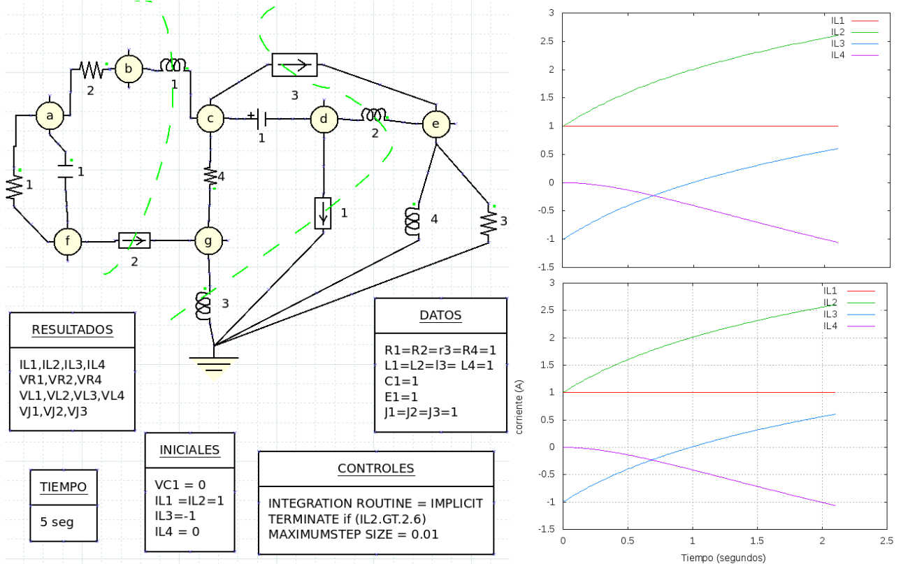
Figura 5: Sistema b. (Izq.): Diagrama y resultados : 2 cut-sets inductivos, en color verde (Der. Arr.:) programa desarrollado (Der. Aba.:) SCEPTRE.
