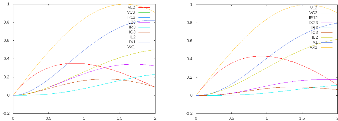
Figura 4: Sistema a. resultados, hasta 2 seg. (Izq.): fuente sinusoidal. (Der.): fuente sinusoidal y bobina “cuadrática”, donde la variación de corriente es proporcional al cuadrado del voltaje y no al mismo.
