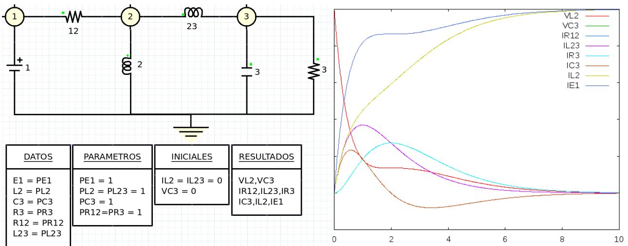
Figura 2: Sistema a. Diagrama del SIMUSOL y resultados, coef. constantes, verificado en (Saravia, 2014).
