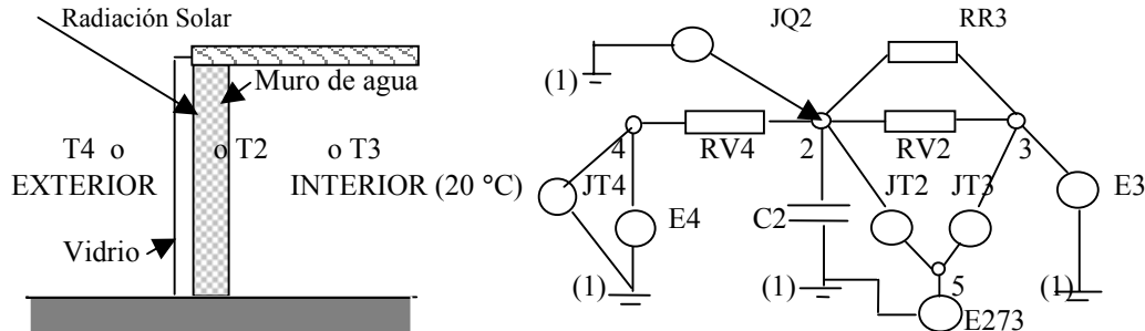
Fig. 1.- Muestra un esquema del sistema térmico a simular, un muro colector de agua, y el circuito análogo.
