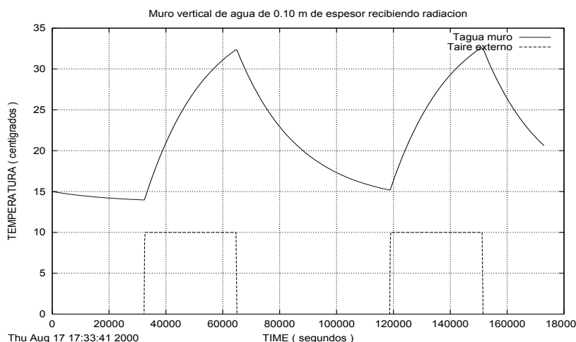
Figura 2.- Resultado de la simulación: temperatura del muro de agua calculada y del exterior (dato).
